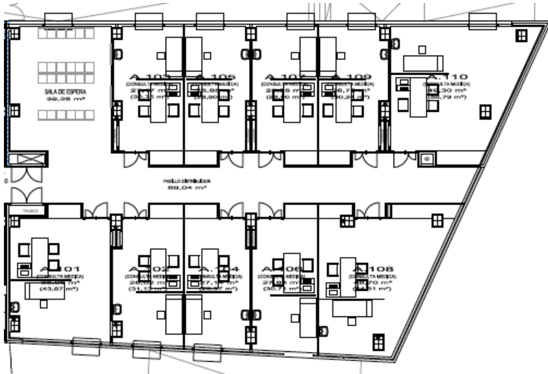
PLANO DE DISTRIBUCION TIPO DE PLANTA
